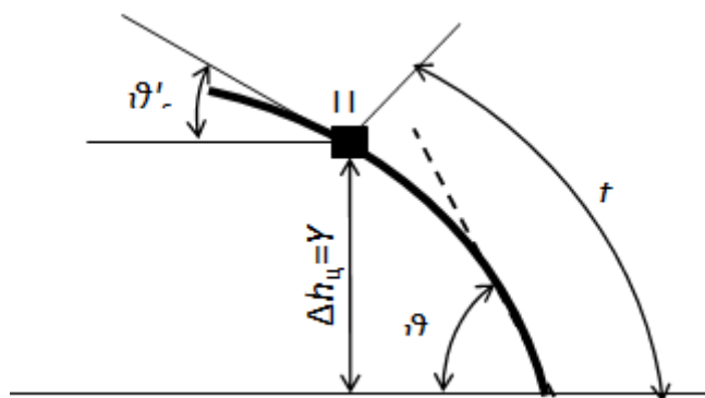
Рисунок 1 – Траектория полета снаряда в районе цели
