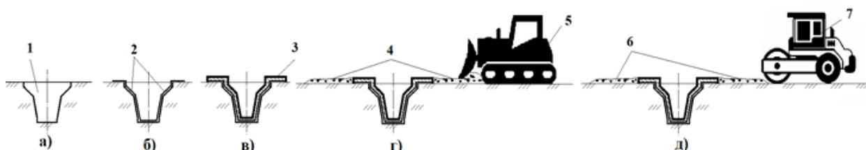
а, б, в - отрывка траншеи, укладка герметичной пленки и установка железобетонных лотков; этап г - подсыпка и разравнивание грунта; этап д - рекультивация и уплотнение грунта на дневной поверхности строительной площадки
