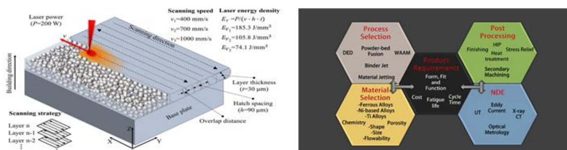
Рисунок 1 – Влияние параметров оборудования на структуру и свойства детали (схема: «параметры процесса – структура – свойства – надежность»).
