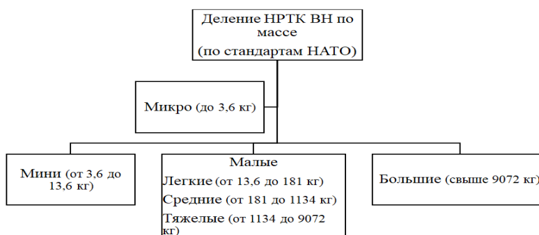
Рисунок 1 – Классификация НРТК стран НАТО по массе
