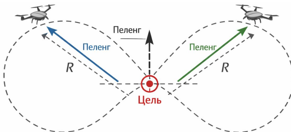
Рисунок 1 – Геометрия траектории полета типа «восьмерка»
