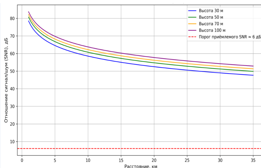
Рисунок 1 – Оценка SNR в зависимости от расстояния
