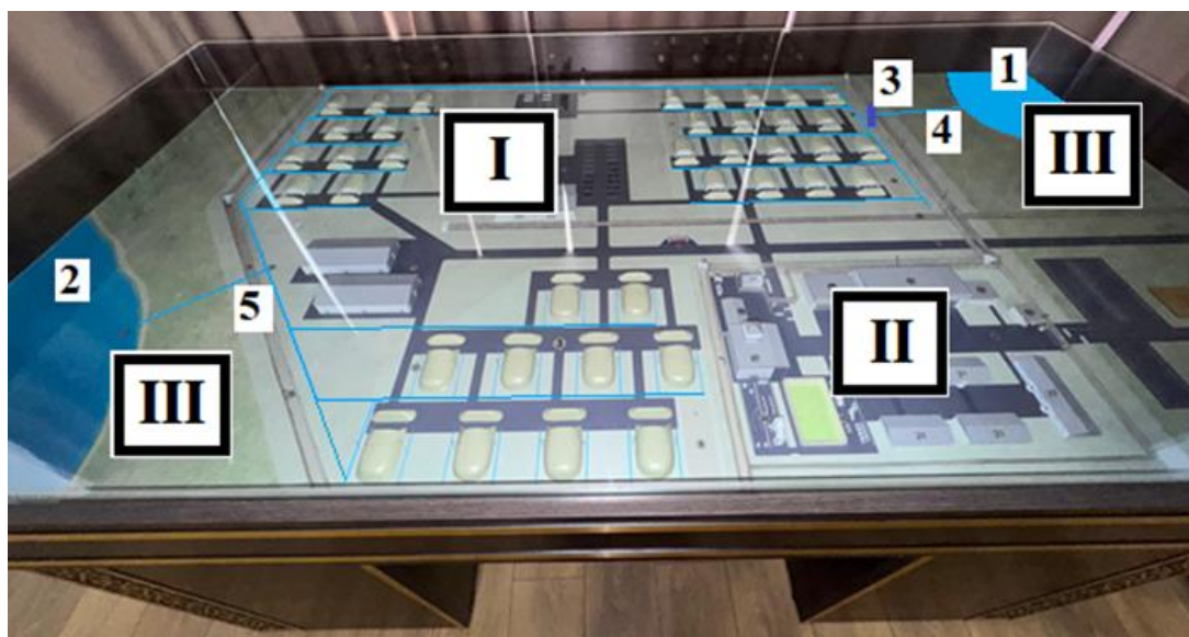
I - техническую территорию базы; II - административно-хозяйственную территорию базы; III - систему сбора и отведения талых и дождевых вод с технической территории базы хранения боеприпасов Рисунок 1 – Модель инфраструктуры базы хранения боеприпасов:
