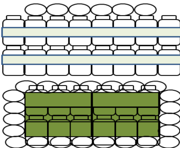
Рисунок 3 – Быстровозводимый каркас из емкостей с водой
